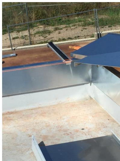
Fixation (Befestigung)
