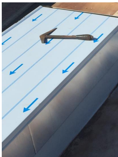
Pose (Verlegen)
